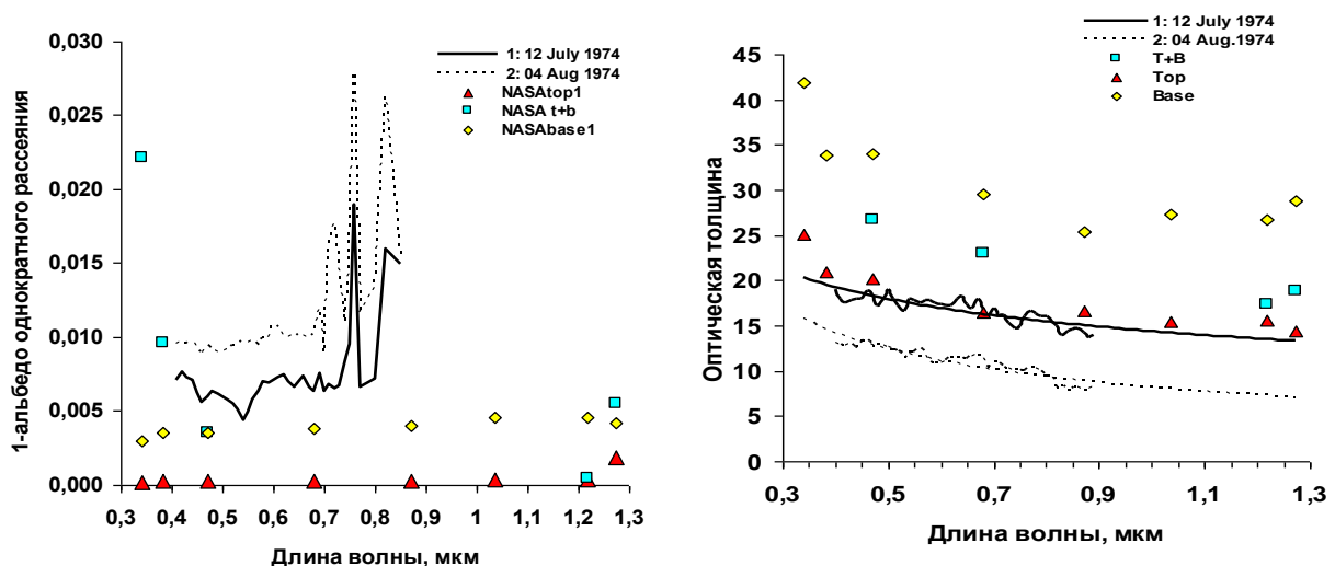
Рисунок 2 – Сравнение спектральных значений оптических параметров полученных из различных самолетных измерений
