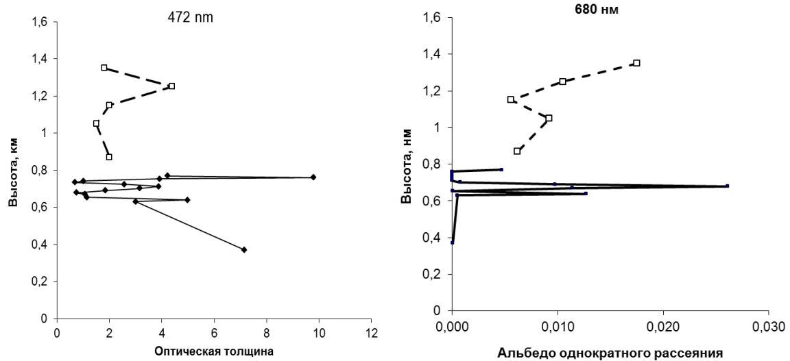
Рисунок 1 – Вертикальные профили а) оптической толщины в канале 472 нм и б) 1-альбеда однократного рассеяния между уровнями измерений в канале 680 нм, восстановленные из измерений NASA в 2000 г. (сплошные линии) и из измерений над Ладогой в 1985 г. (штриховые линии)
